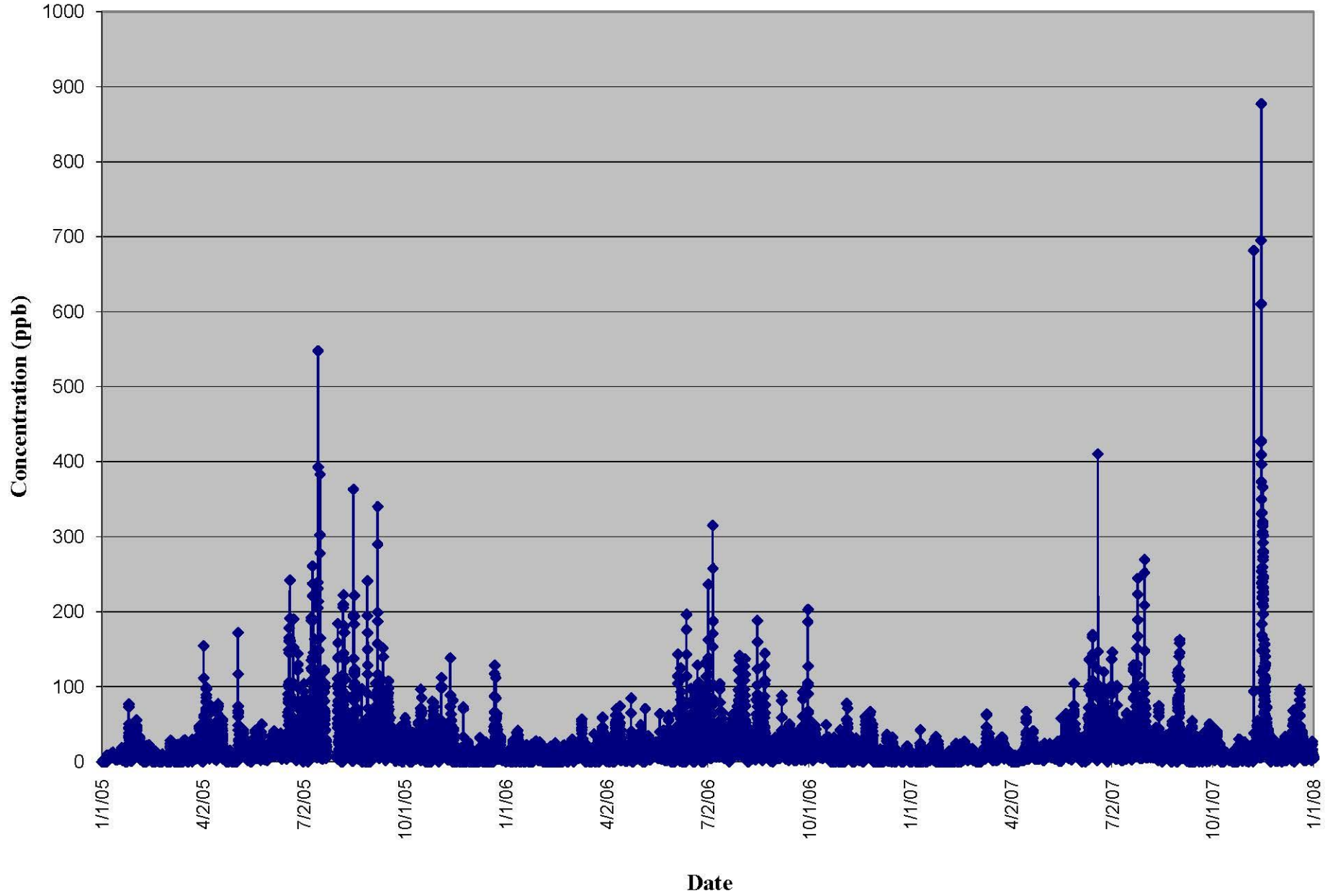
Kanawha CAFO: Ammonia vs Time (2005-2007)
