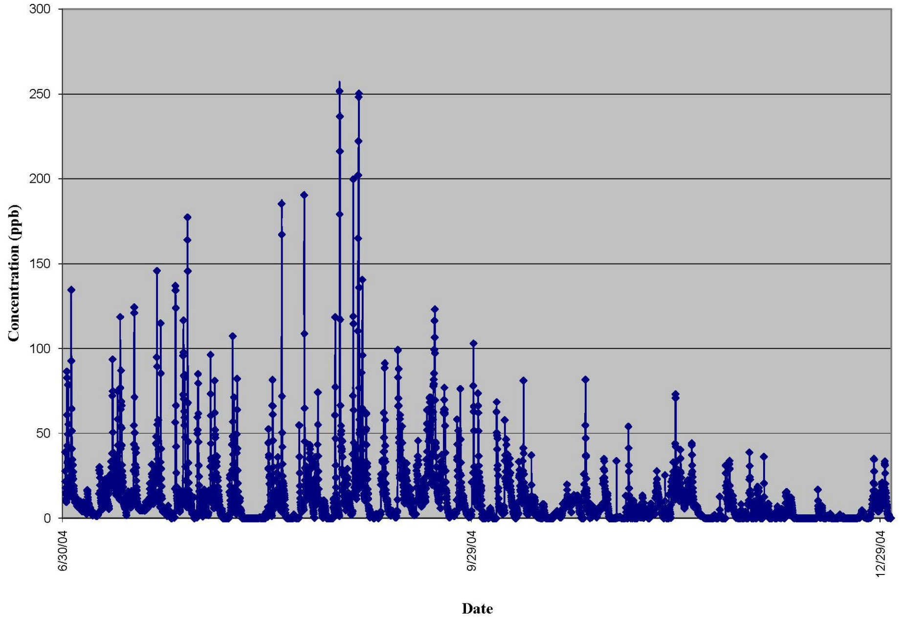
Kanawha CAFO: Ammonia vs Time (2004)
