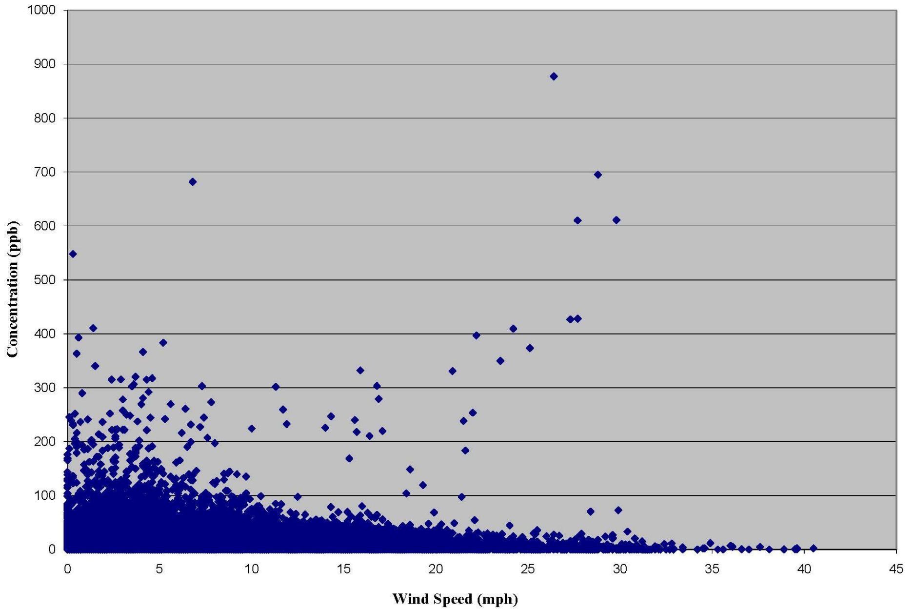
Kanawha CAFO: Ammonia vs Wind Speed (2004-2007)
